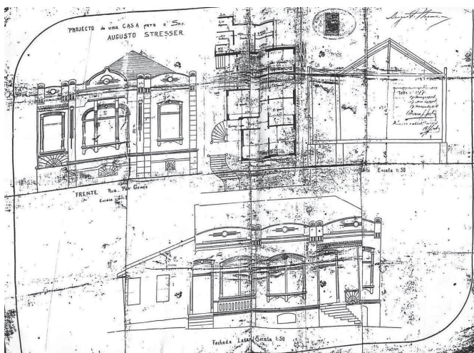
Figura 7 - Planta arquitetônica da casa elaborada por Augusto Stresser
